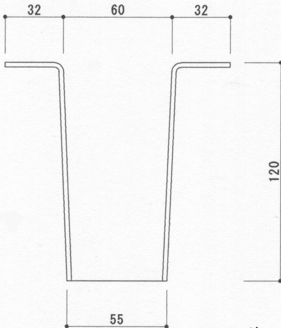
FRPドレンI型
